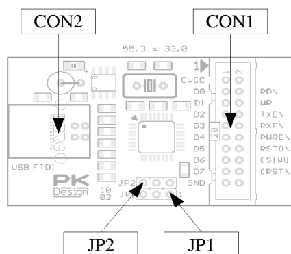
Obr. 1 - umístění konektorů a propojek
