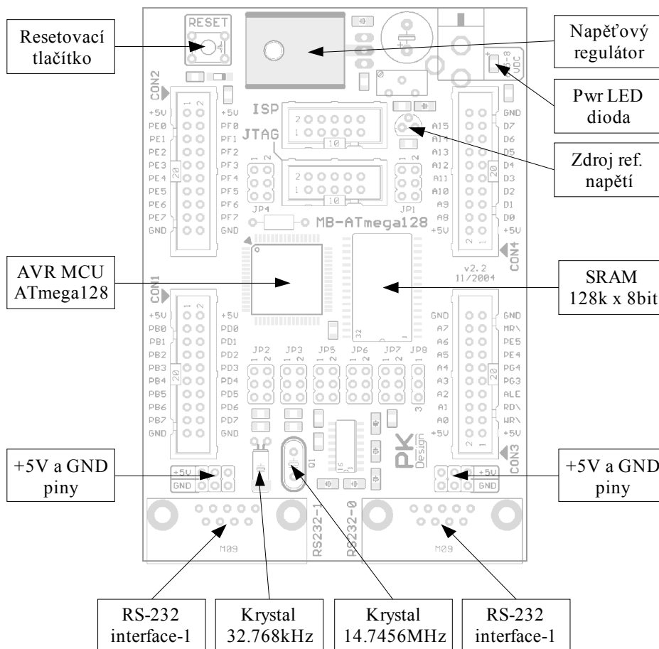
Obr. 1 - periferie základové desky
