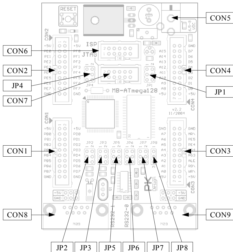
Obr. 2 - rozmístění konektorů a propojek na základové desce
